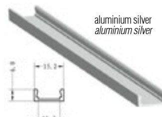
PERFIL Aluminium DE SUPERFICIE PARA LEDS 2000 x 15 nº2
